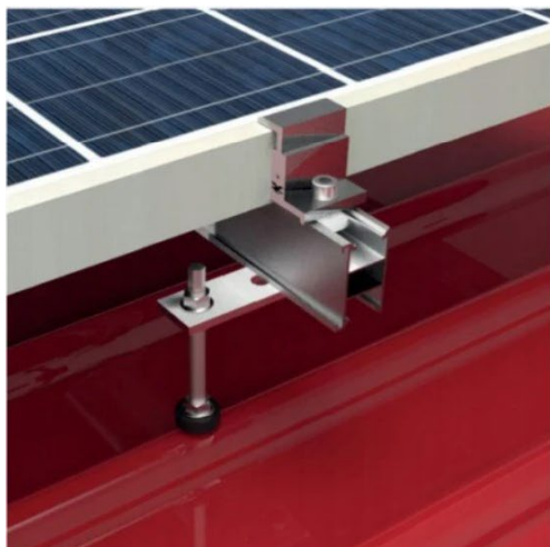
□ Foto structură montaj tip tablă
