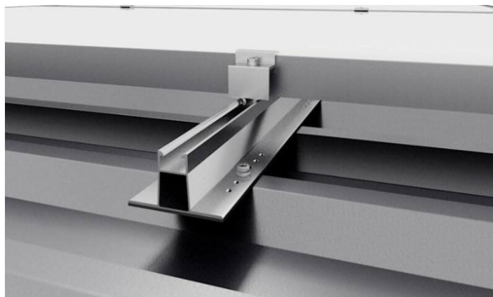
□ Foto structură de montaj tip hală - panouri sandwich
